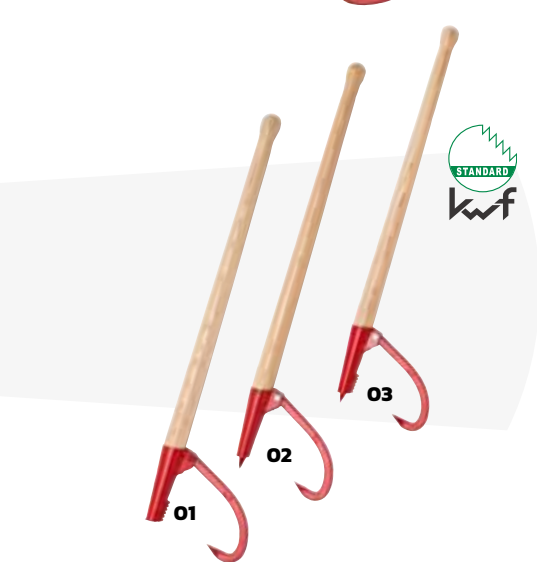
Wendehaken , mit Eschenstiel Cant hook , ash handle Crochet de manutention , manche frêne Gancio giratronchi , manico frassino
